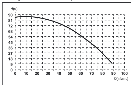
БЦПЭ-ГВ-75-0,8-65
