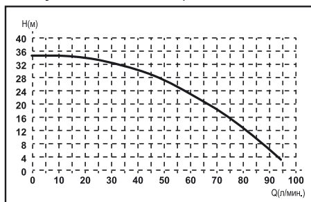
БЦПЭ-ГВ-100-0,8-28
