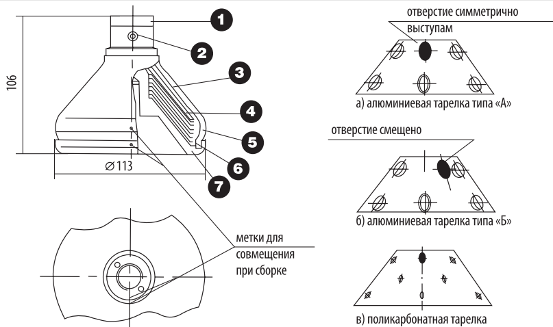
Рисунок 3. Барабан
